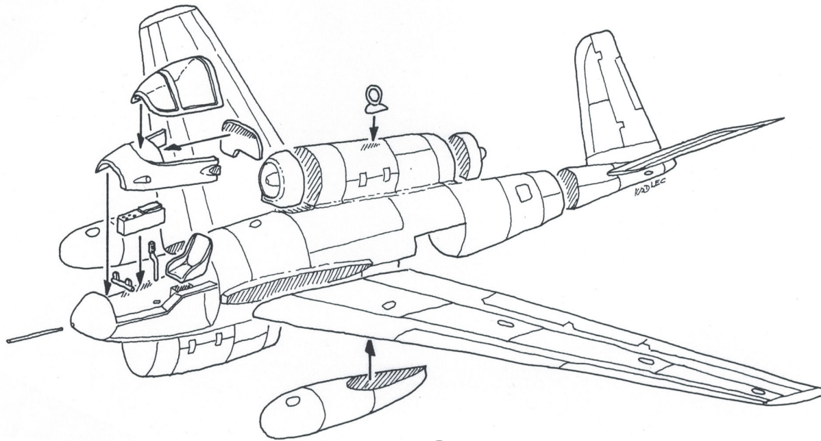
Heinkel P.1079 A
